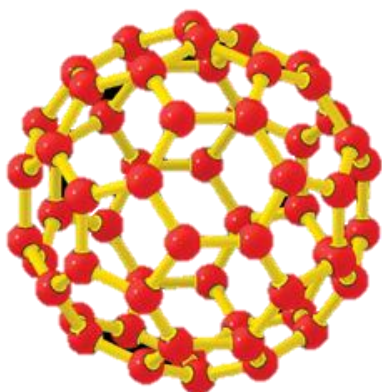
Fulerenă C 60
