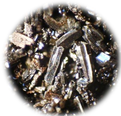
Fulerene în formă cristalină
